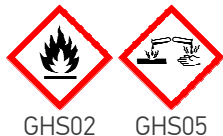
GHS02 GHS05
